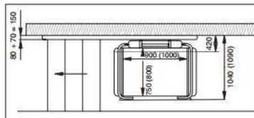
Målskitse: plantegning, alle mål i mm.
