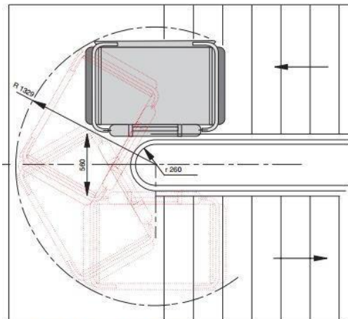
Eksempel: platformlift 750x900, alle mål i mm.
