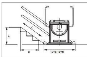
Målskitse: opstalt, alle mål i mm. Diameter på skinne: 90 mm
